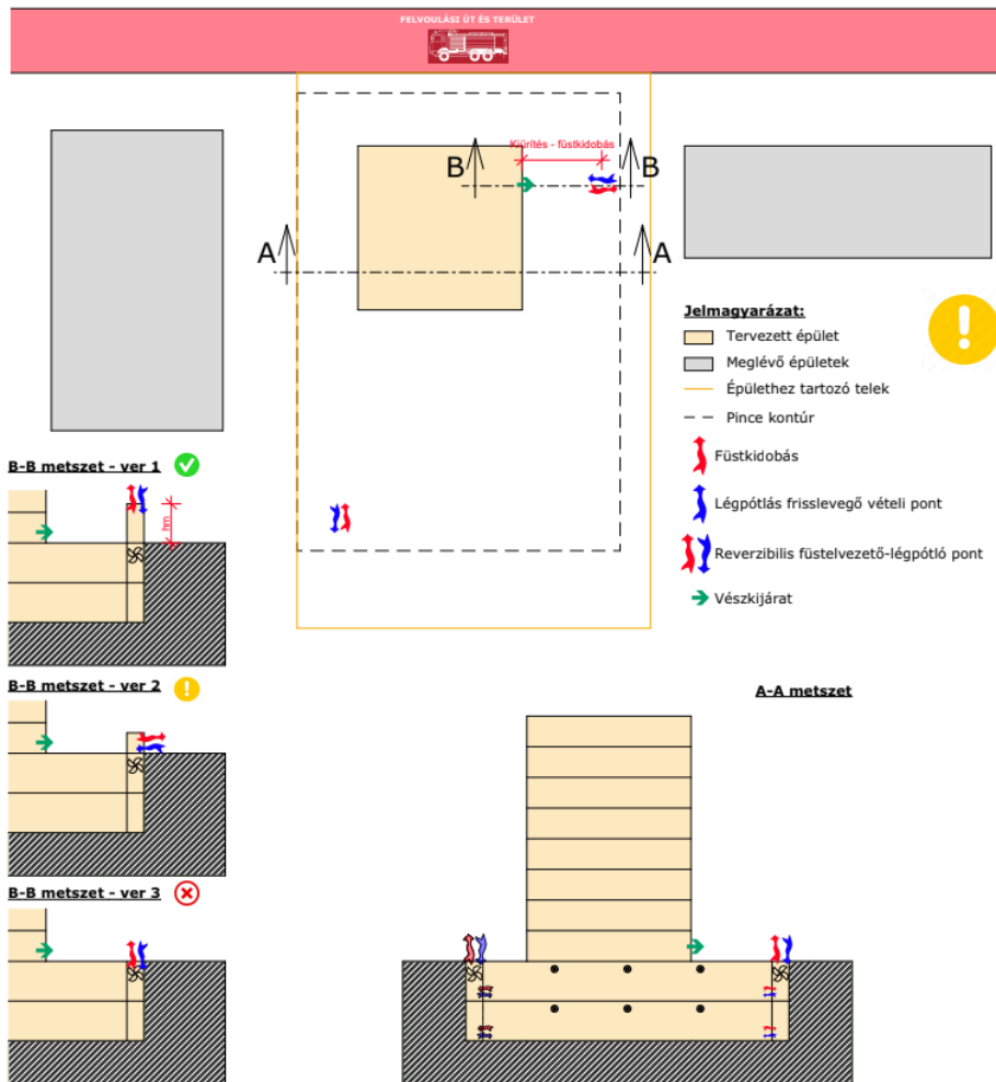
U.6. ábra: Ritka, szabadon álló beépítés esetén részletes átgondolást igénylő megoldások (vész)kijárat közelében
