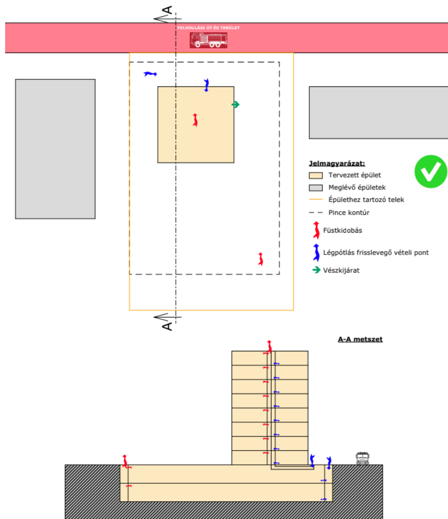
U.4. ábra: Ritka, szabadon álló beépítés esetén javasolt jó megoldások
