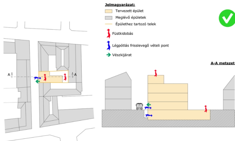
U.1. ábra: Sűrű városi beépítés esetén javasolt jó megoldások
