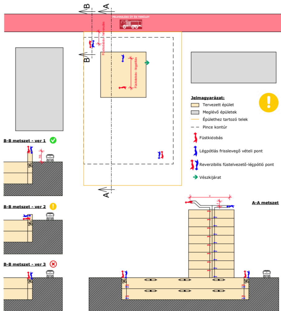
U.5. ábra: Ritka, szabadon álló beépítés esetén részletes átgondolást igénylő megoldások tűzoltási felvonulási terület közelében
