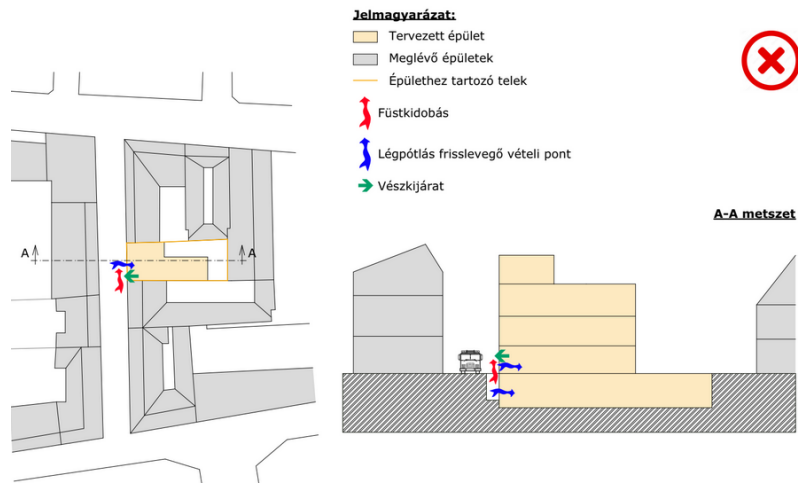
U.2. ábra: Sűrű városi beépítés esetén nem megfelelő megoldások
