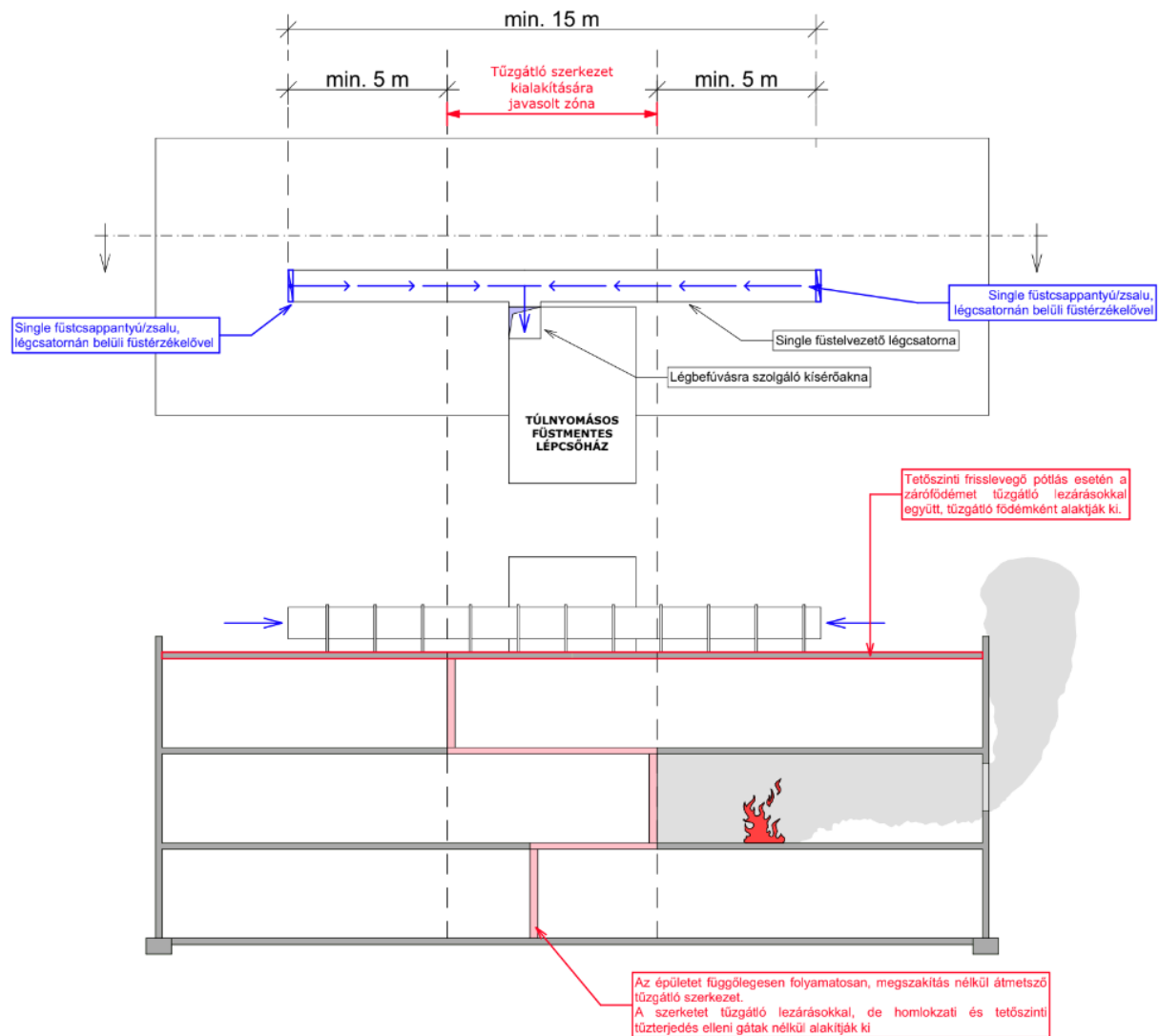
5H-6. ábra: Példa túlnyomásos füstmentes lépcsőház tetőszintről történő frisslevegő ellátása esetén a frisslevegő vételi pontok javasolt elhelyezésére
