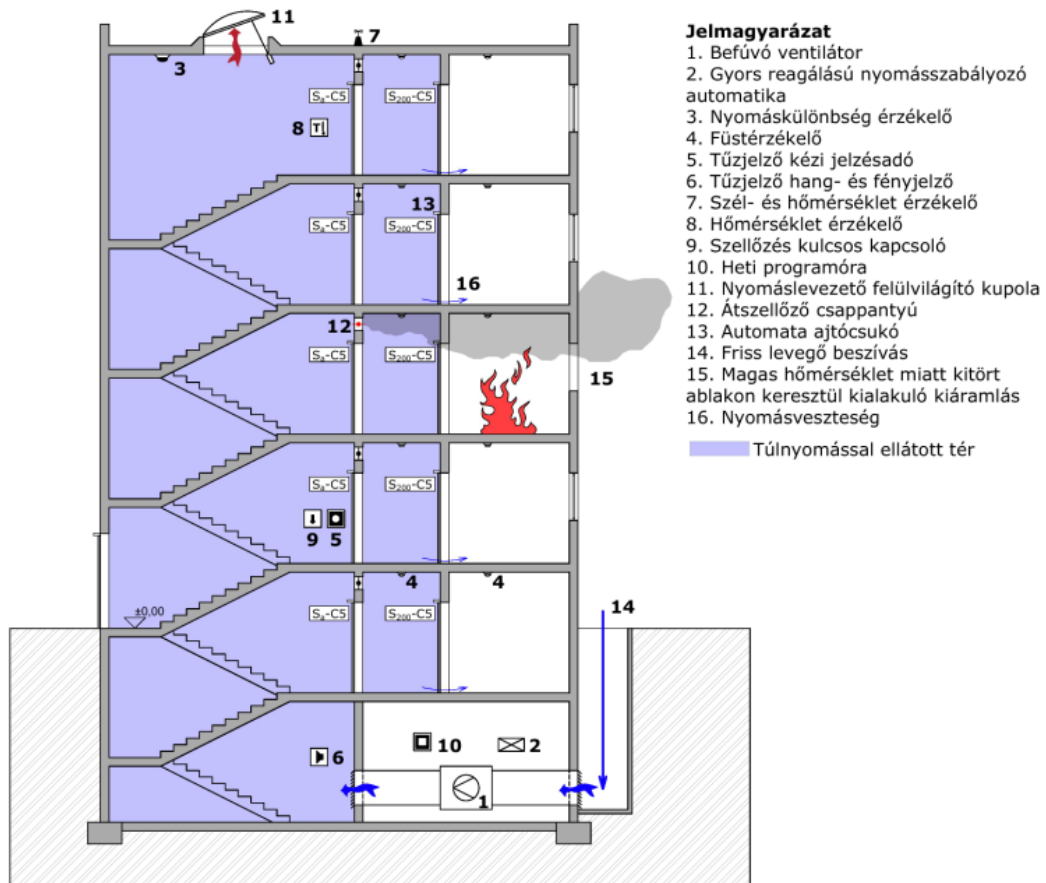
H-2. ábra: Példa előteres túlnomásos füstmentes lépcsőház kialakítására, szabályozott üzemű ventilátorral, túlnomás levezető kupolával
