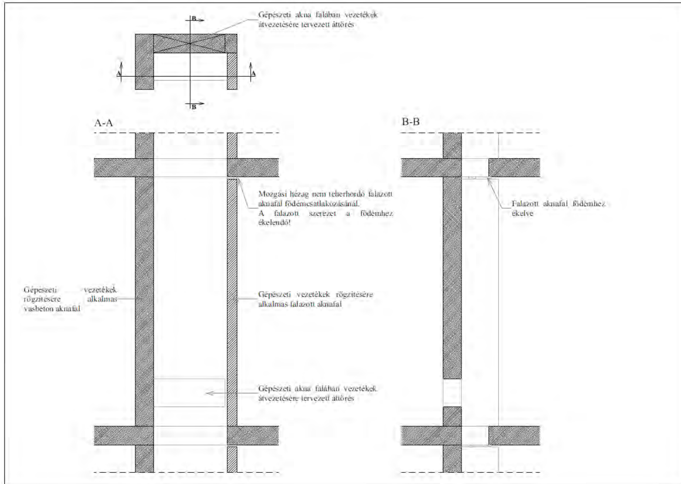
L/I.1. ábra - Szerelőakna szerkezetkész állapotban, a gépeszeti és villamos szerelés megkezdése előtt
