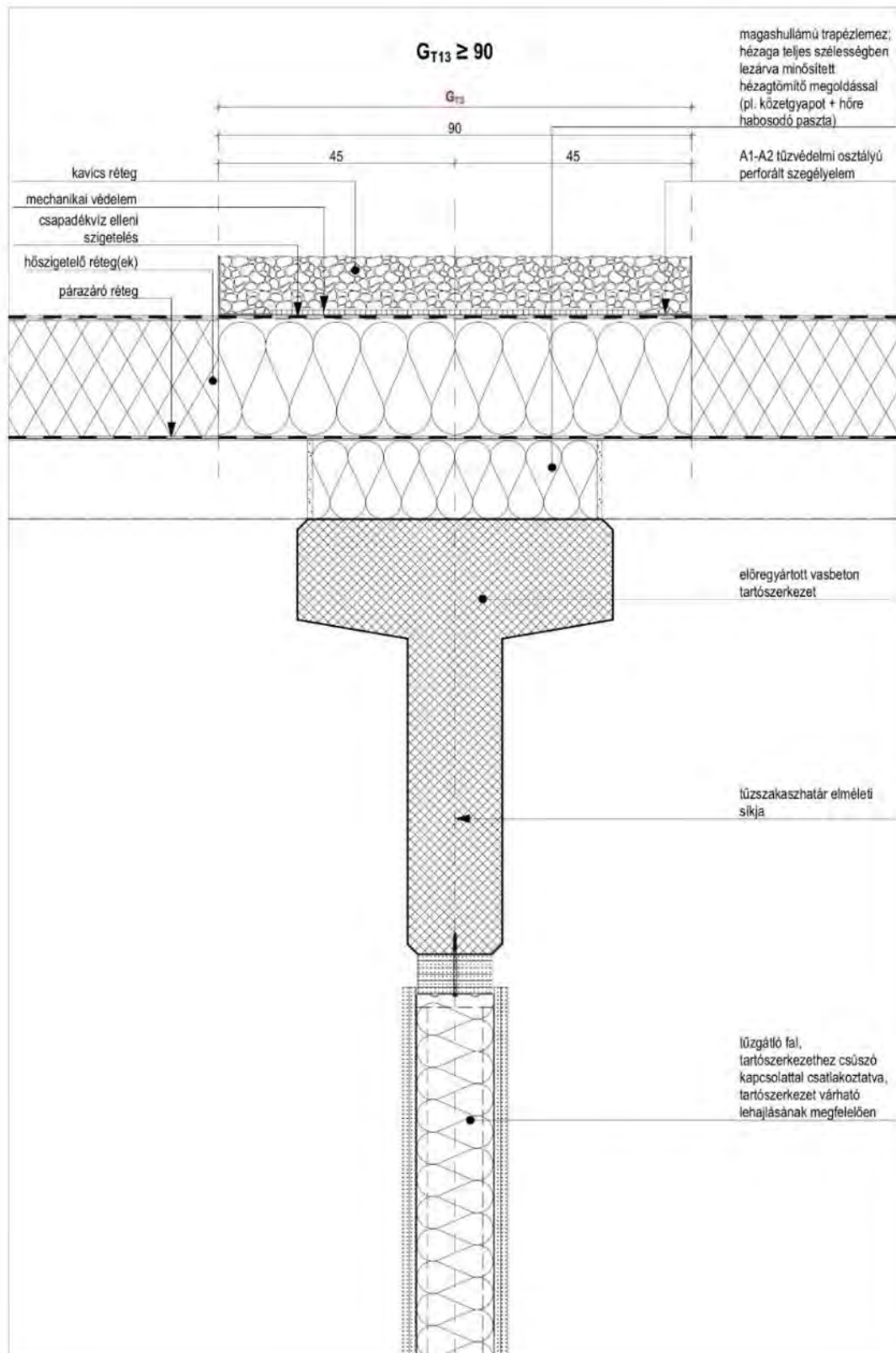
3F8 sz. ábra: előregyártott vasbeton vázszerkezetű és könnyű tetőfödém térelhatároló szerkezetű épület tűszakaszhatárához kapcsolódó síkban tartott tetőszintű tűzterjedés elleni gátjának példája
