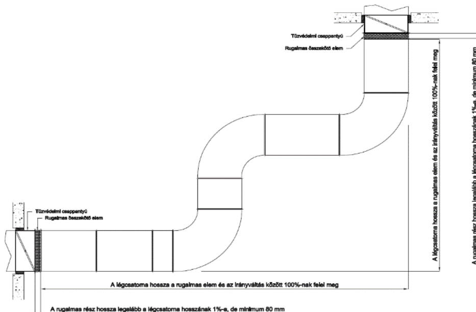
2D5.1.7. ábra. Acél szellőző légszatórna több irányváltással két tűzcsappantyú között rugalmas összekötő elemek alkalmazásával
