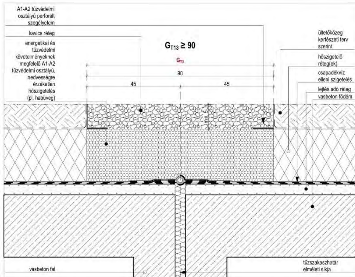
3F7 sz. ábra: extenzív zöldtető tetősíkban tartott tetőszinti tűzterjedés elleni gátja kialakításának példája
