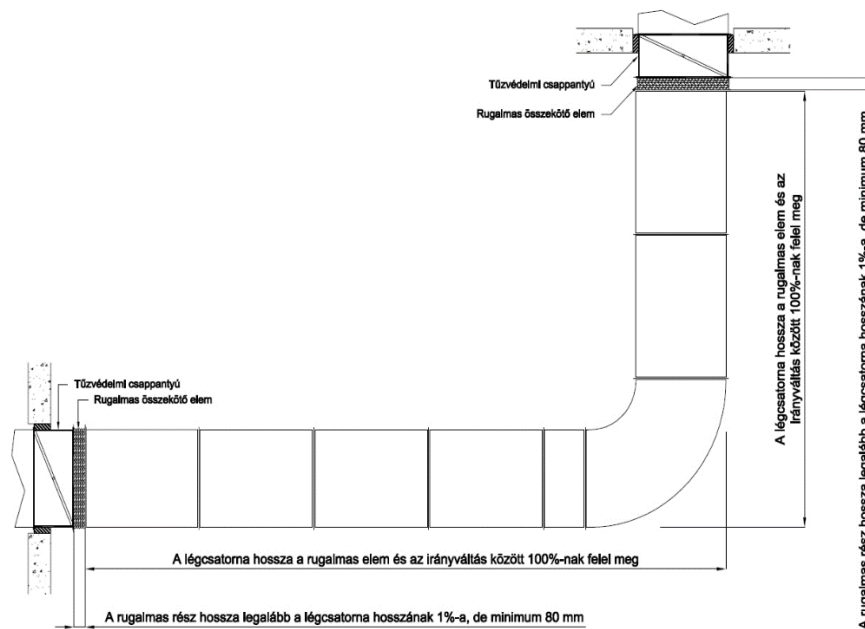
2D5.1.6. ábra. Acél szellőző légszatórna irányváltással két tűzcsappantyú között rugalmas összekötő elemek alkalmazásával
