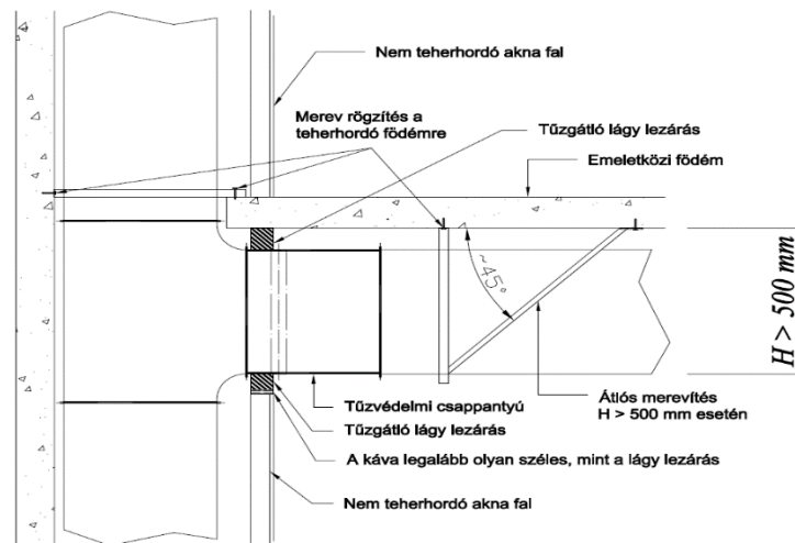
2D5.3.5. ábra. Nem teherhordó aknafalba épített nagy méretű csappantyú a födémhez és az akna teherhordó falához mereven rögzített légcsonnákkal
