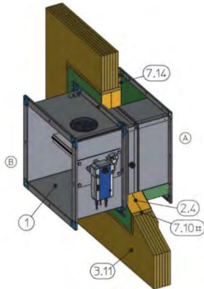
3D5.6.7. ábra. Tűzgátló csappantyú száraz (lágý lezárásos) beépítése CLT fal síkján belül
