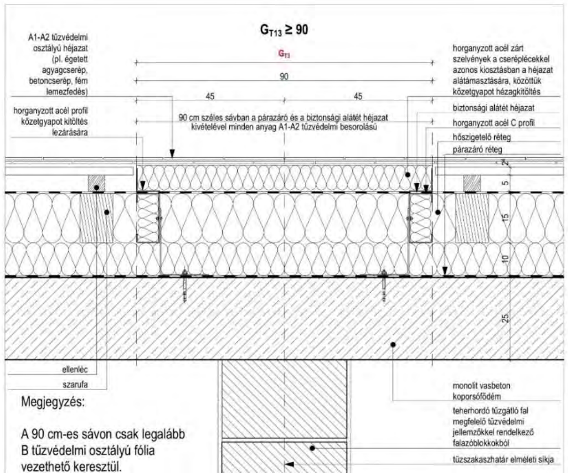
3F5 sz. ábra: magastető tetősíkban tartott tetőszinti tűzterjedés elleni gátja kialakításának példája, vasbeton koporsófödém esetén
