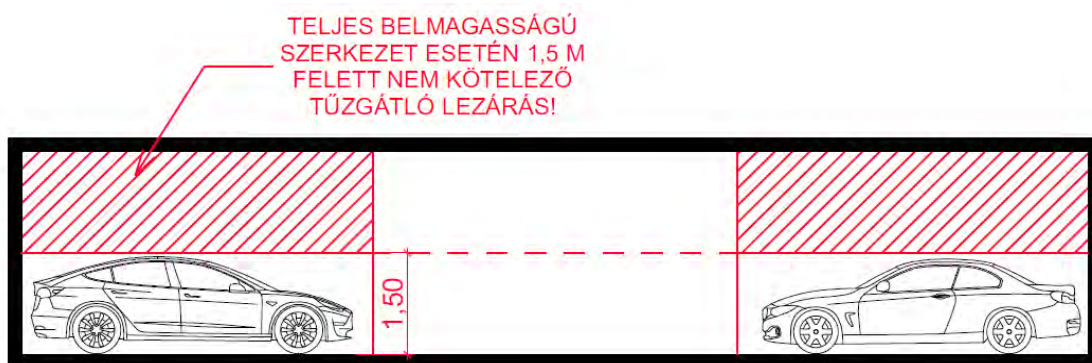
23. ábra – Teljes belmagasságú fix leválasztásra vonatkozó feltétel
