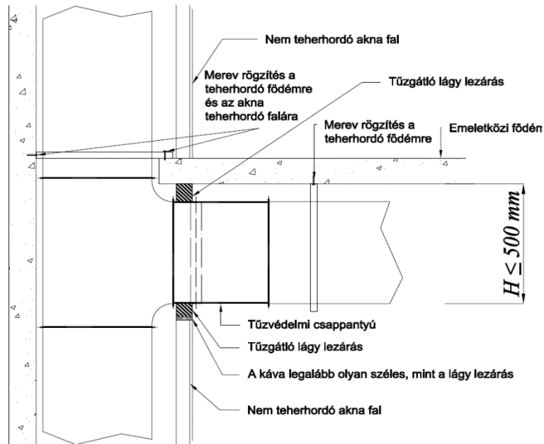
2D5.3.4. ábra. Nem teherhordó aknafalba épített kis méretű tűzvédelmi csappantyú a födémhez és az akna teherhordó falához mereven rögzített légcsonnákkal
