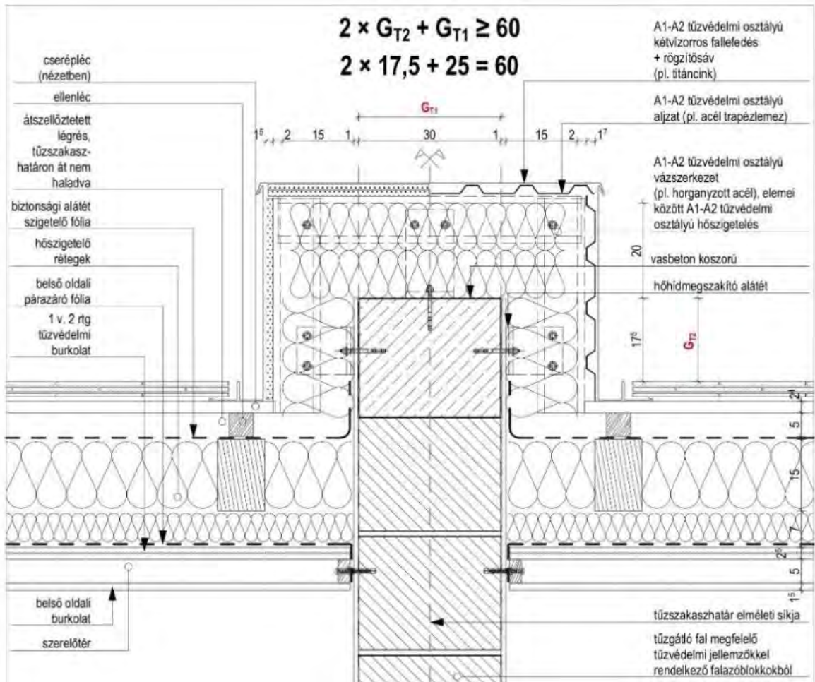
3F3 sz. ábra: magastető tetősíkból kiemelkedő tetőszintű tűzterjedés elleni gátjának példája
