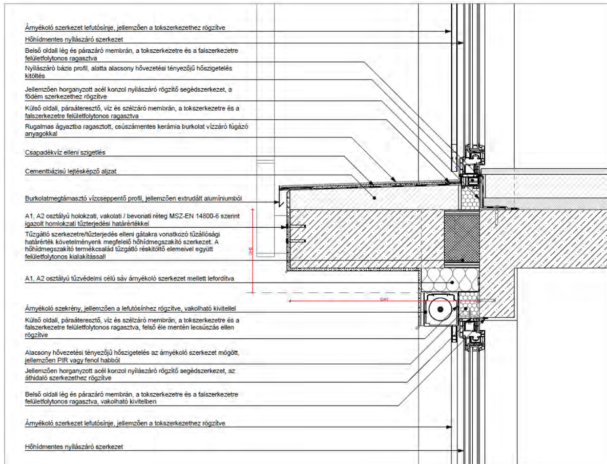
4F18 sz. ábra. Homlokzati tűzterjedés elleni gát geometriai értelmezése hőhíd megszakítóval erkély esetén
