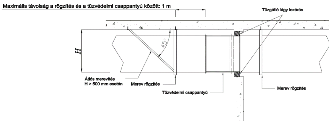
2D5.3.1. ábra. Tűzcsappantyú és mereven rögzített acél légszatóna kapcsolódása rugalmas összekötő elemek nélkül
