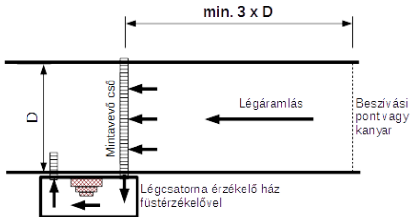
7. ábra Légszatórna érzékelő elhelyezkedése
