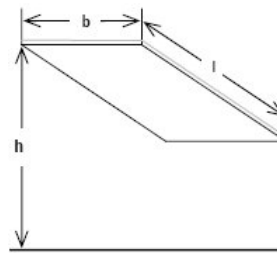
4. ábra Szintosztó födém adatainak magyarázata
